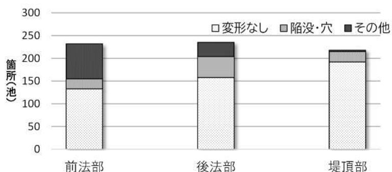
堤体の変形状況(R3~R5)
